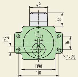
带耳减速箱
