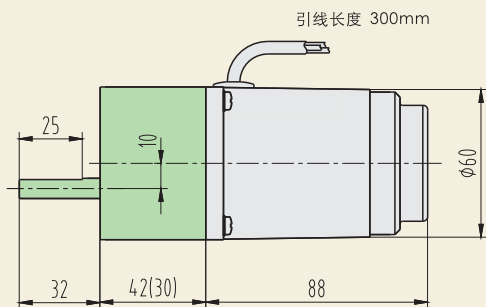
( )尺寸为速比≤18的尺寸
