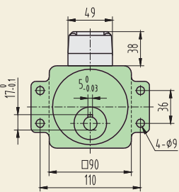
带耳减速箱
